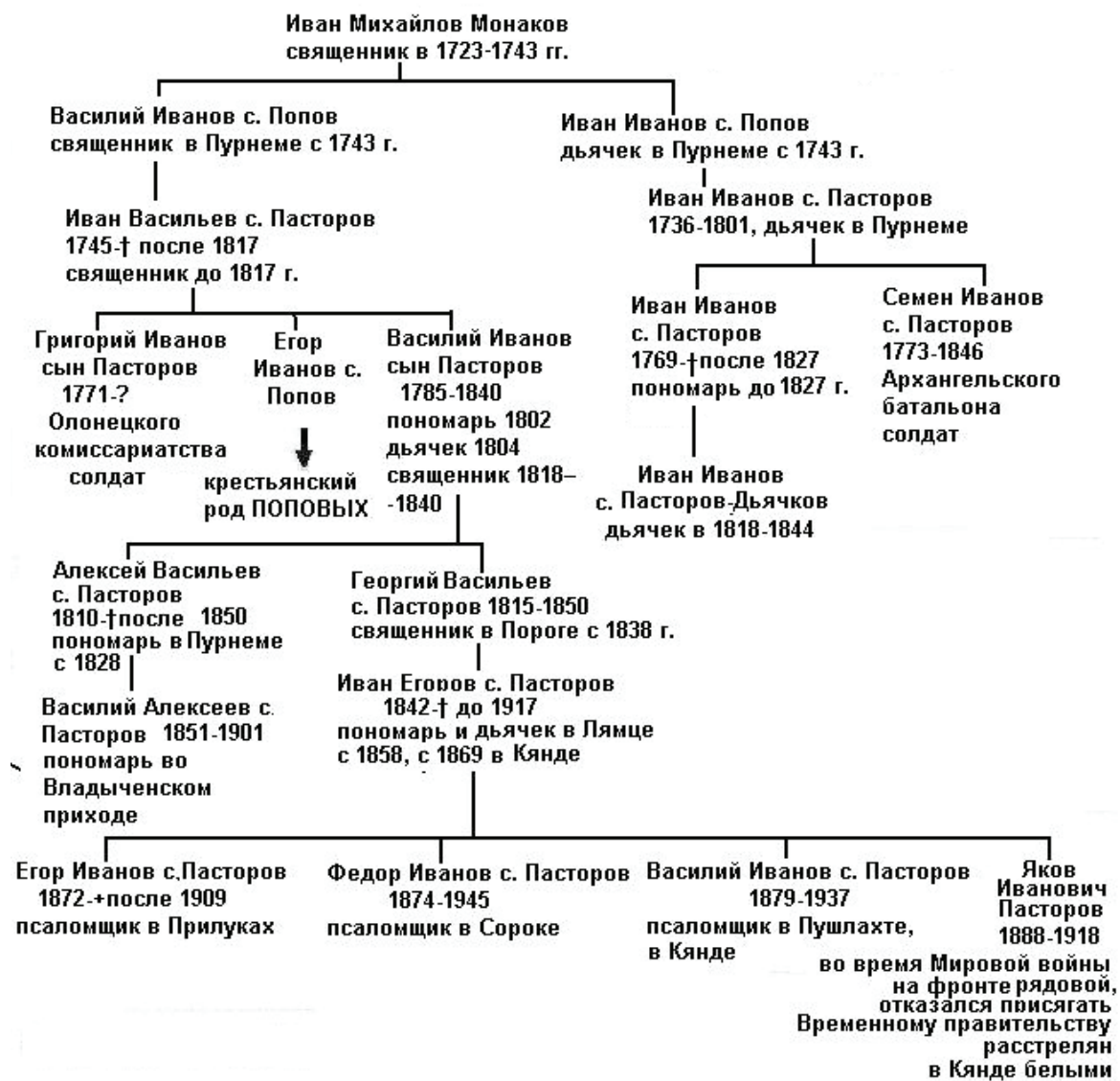
Рисунок 3. Сокращенная схема родства Пасторовых – священников, дьячков, пономарей и псаломщиков в церквях Архангельской губернии в XVIII-XX вв.
